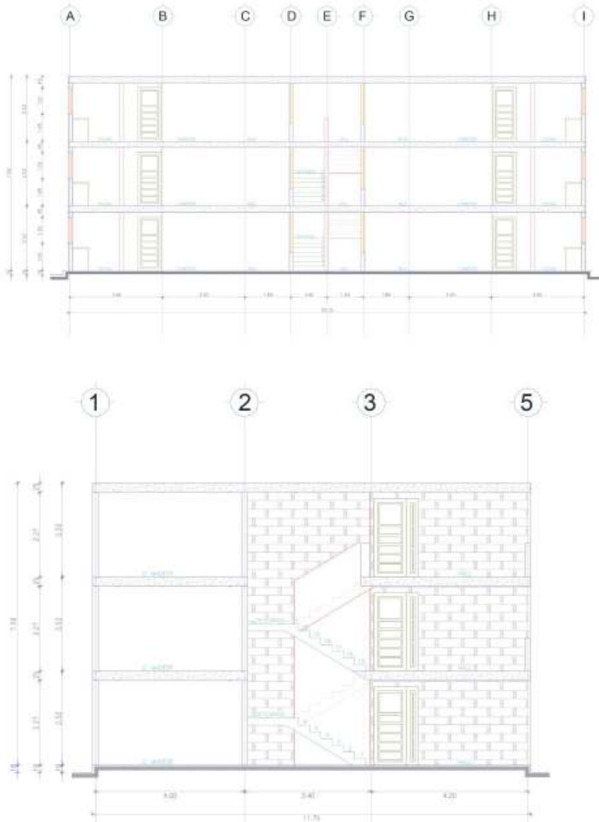
Figura 47: Vivienda en consideración
