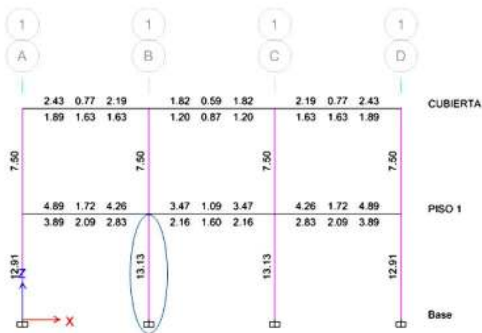
Figura 28: Resultados del análisis estructural para diseño a Flexo – Compresión (Acero de Refuerzo en cm²)
