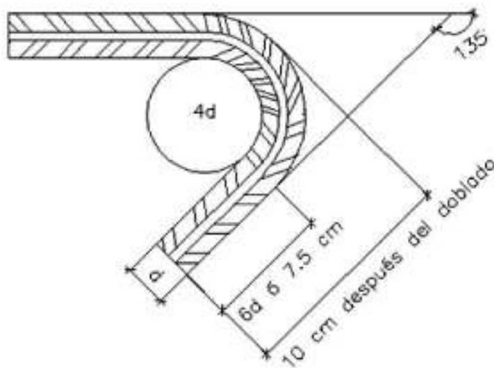
Figura 9: Geometría del gancho longitudinal de doblado de estribos de 8 mm
