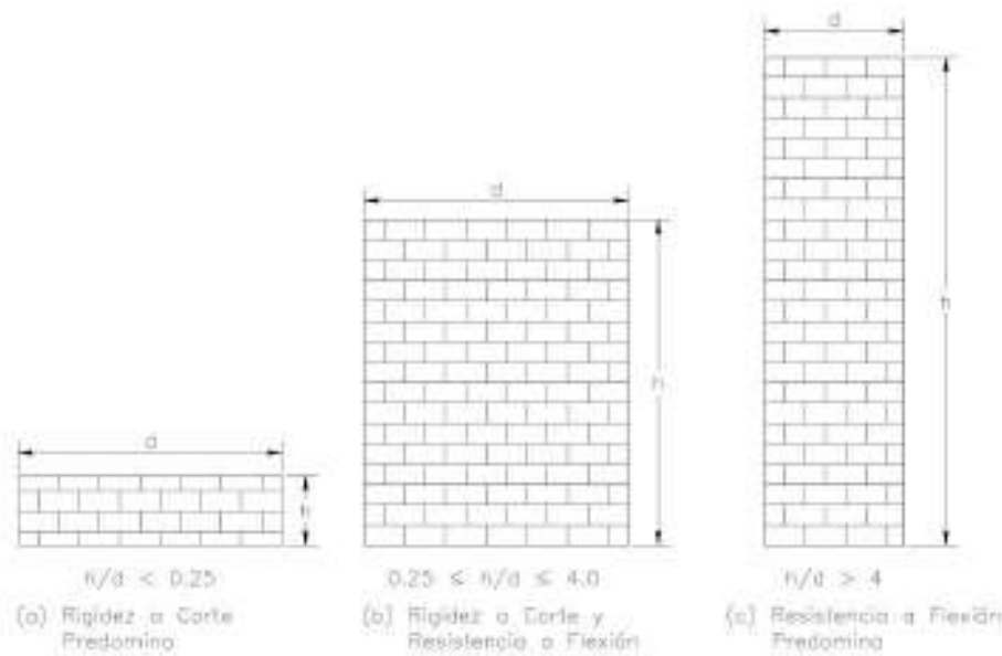
Figura 56: Filosofía general del diseño para la resistencia de mampostería confinada
