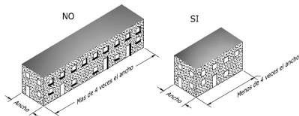
Figura 3: Relación de aspecto, largo/ancho en edificaciones
