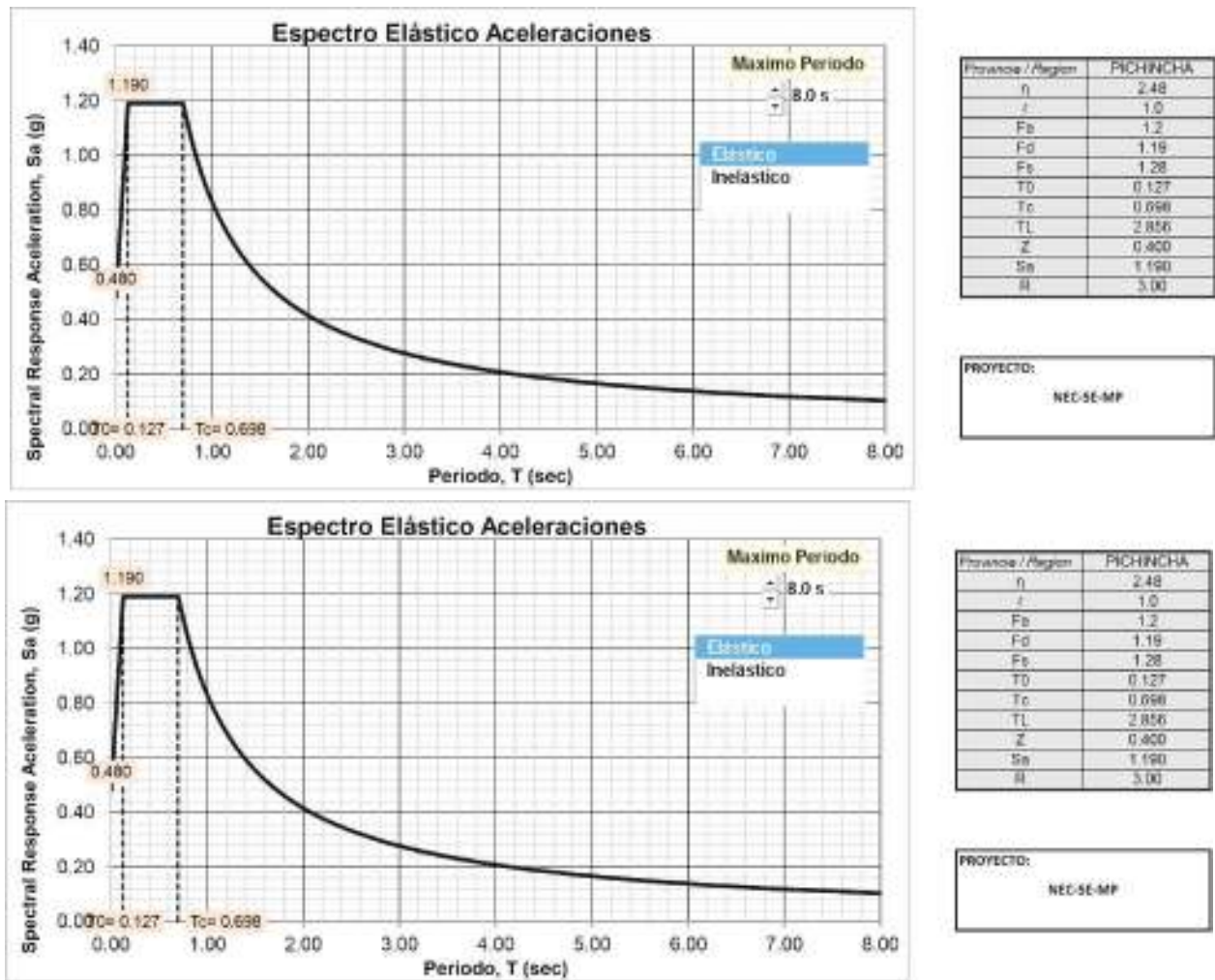
Figura 37: Espectro elástico de aceleraciones
