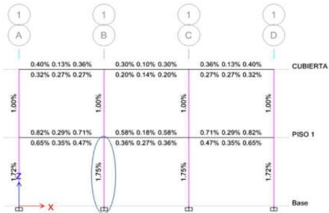
Figura 29: Resultados del análisis estructural para diseño a Flexo – Compresión (Cuantía Requerida)
