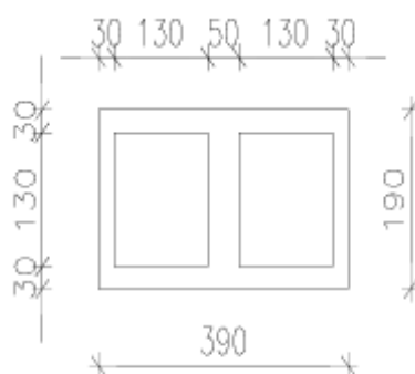
Bloque HS 190x390x190 Dimensiones en mm Resistencia 7MPa
