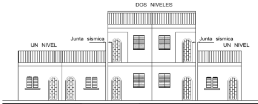
Figura 7: Elevación (c), Ubicación esquemática de las juntas sísmicas de unidades habitacionales multifamiliares
