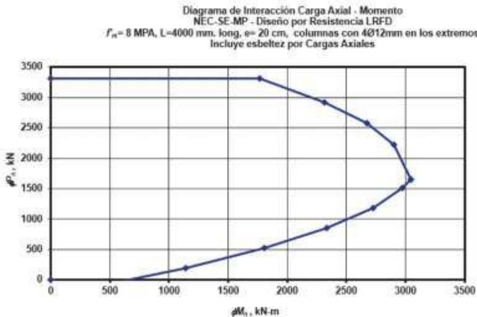
Figura 59: Cálculo del diagrama de interacción para el muro de mampostería confinada
