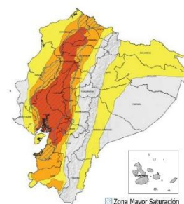
Estimación de Precipitación Pronosticada
