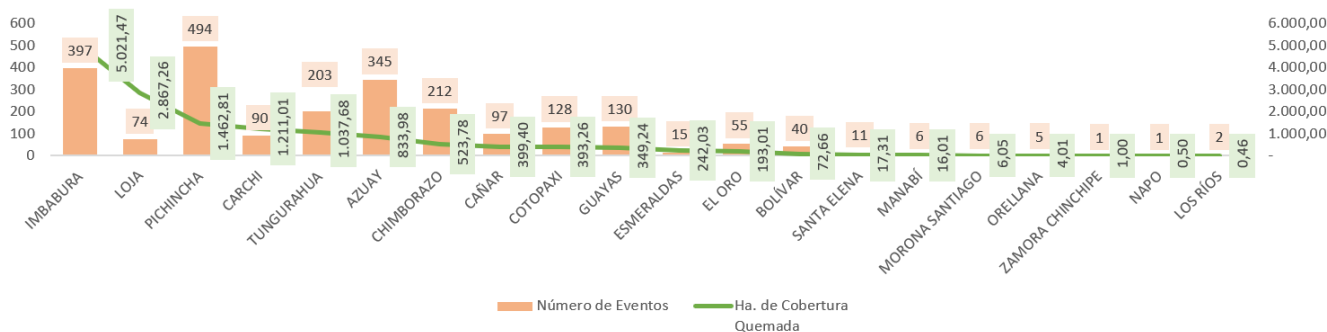
Nro. Incendios Forestales vs Ha. de Cobertura Vegetal Quemada
