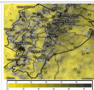
Fig. 2. Previsión de la distribución de la cobertura nubosa. Fuente: Modelo GEM – Meteologix.
