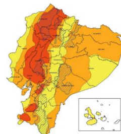
Estimación de la Precipitación Pronosticada
