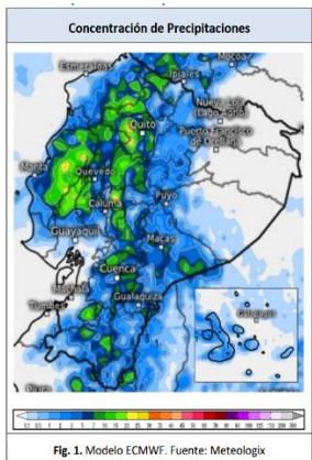
Fig. 1. Modelo ECMWF. Fuente: Meteorología
