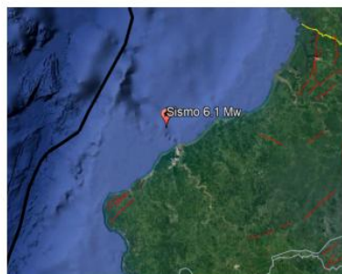
Figura 1.a. Mapa de Localización del evento registrado a las 06H44 (TL).
