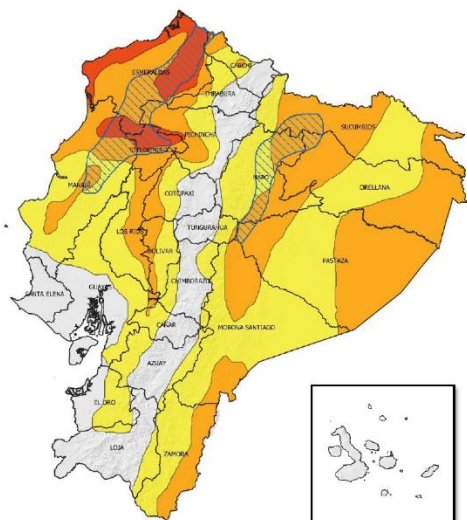
Estimación de Máxima Precipitación Acumulada Diaria
