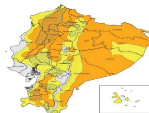
Estimación de Máxima Precipitación Acumulada Diaria
