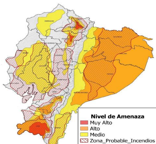
Fig. 1: Mapa de nivel de amenaza: Incremento de temperatura durante el día y zonas favorables a incendios forestales.
