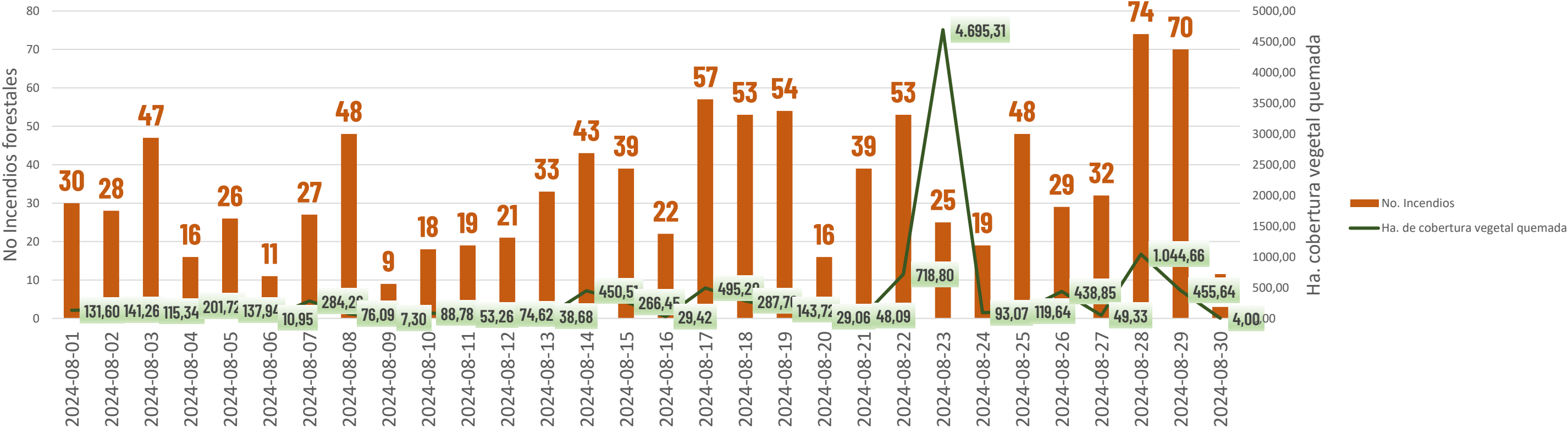
No. de incendios forestales vs ha. quemada regsitrado en el mes de agosto, desagregado por días
