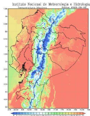
Temperatura Máxima
