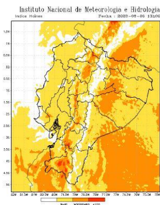
Índice HAINES
