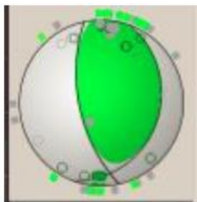
Figura 1.b. Mecanismo Focal obtenido con inversión de formas de onda (SC3). La magnitud resultante con este método es 4.5 Mw (magnitud momento).
