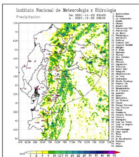
Figura 1.- Estimación de precipitación acumulada en base al modelo WRF - INAMHI
