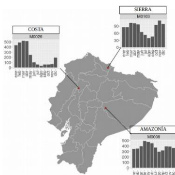
Figura 1: precipitación media mensual del periodo 1986-2018 para 3 estaciones representativas que tienen la mayor cantidad de información
