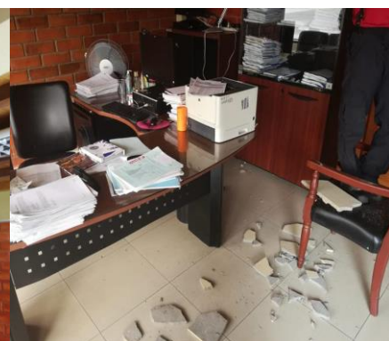
Morona Santiago – Afectación a la mampostería de la Fiscalía General del Estado Gualaquiza
