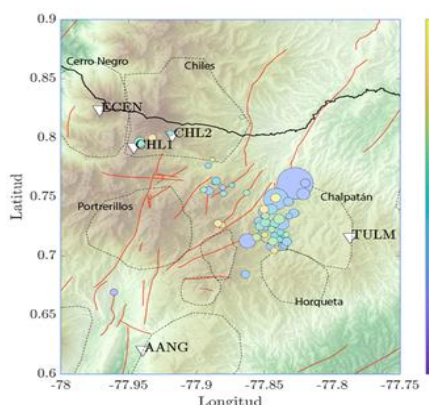
Figura 2: Localizaciones de eventos de la madrugada de hoy en la provincia de Carchi. El tamaño del símbolo en estas figuras es proporcional a la magnitud del evento
