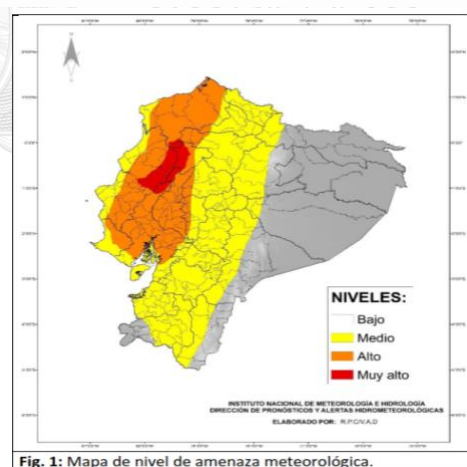
Fig. 1: Mapa de nivel de amenaza meteorológica.
